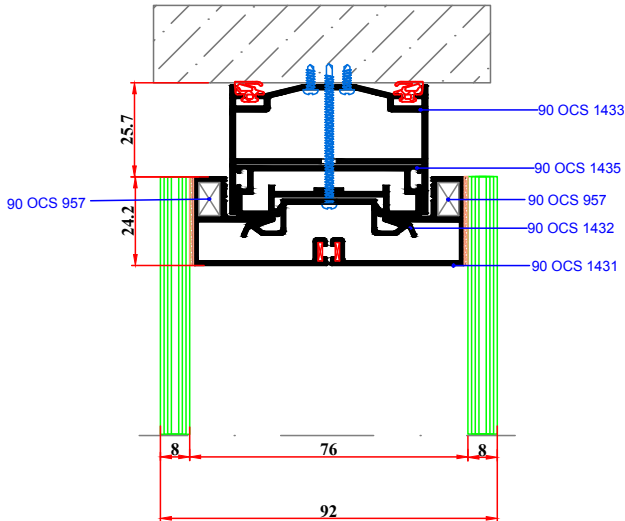
2 NOLU DETAY
